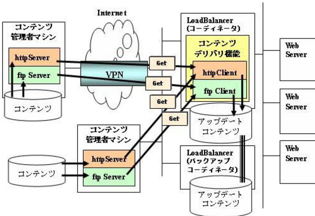
システム構成例 2
