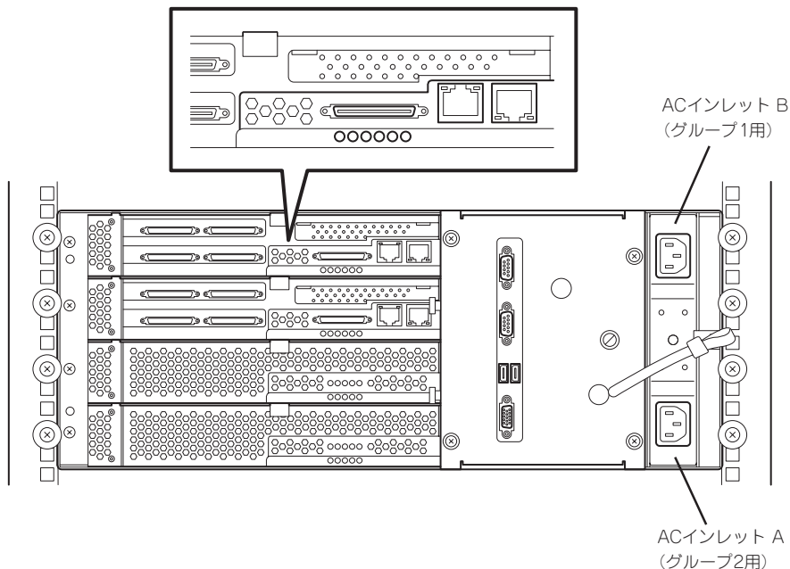
ラックマウントモデル
