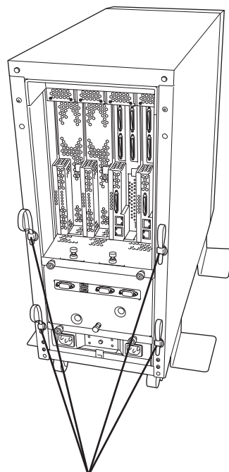
丸印の部分にあるケーブルタイで固定する (ケーブルタイは筐体に添付されています)
