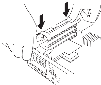
ロープロファイルタイプ
