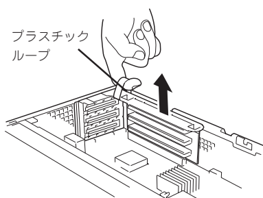
ロープロファイルタイプ
