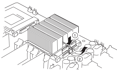
オプションのCPUの場合 (マイナスイヤクリップをワイヤクリップに差し込んで取り外す)
