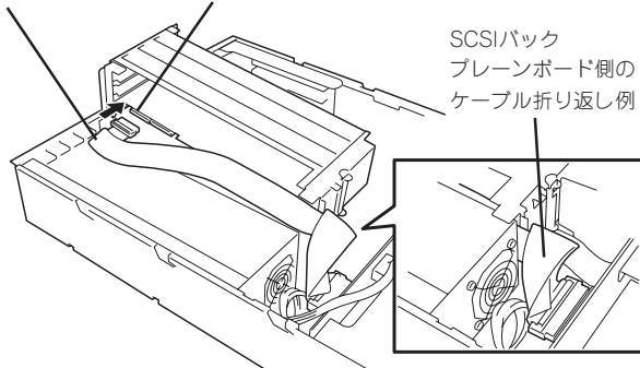
フルハイトタイプの場合
