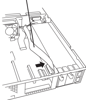
マザーボード側のケーブルの取り外し
