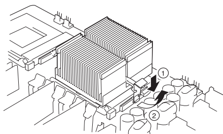
標準装備のCPUの場合 (指でクリップを押して金具を取り外す)
