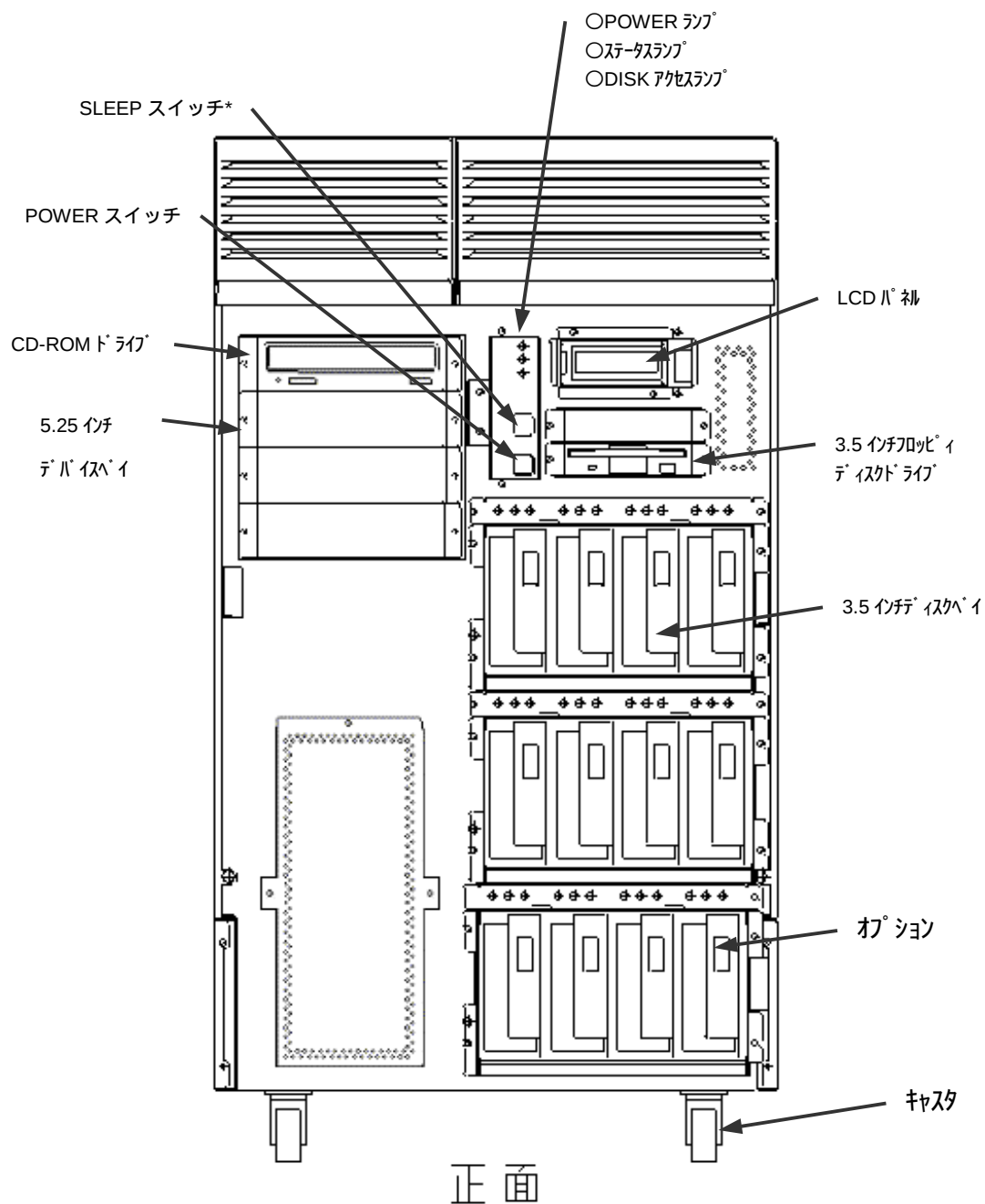
正面図
