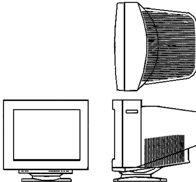
(N8571-10) 筐体寸法 498mm(W)×474mm(D)×505mm(H)
