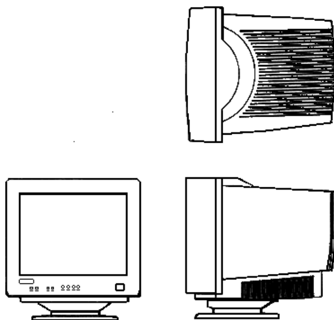
(N8571-11) 筐体寸法 368mm(W)×406.5mm(D)×382.5mm(H)
