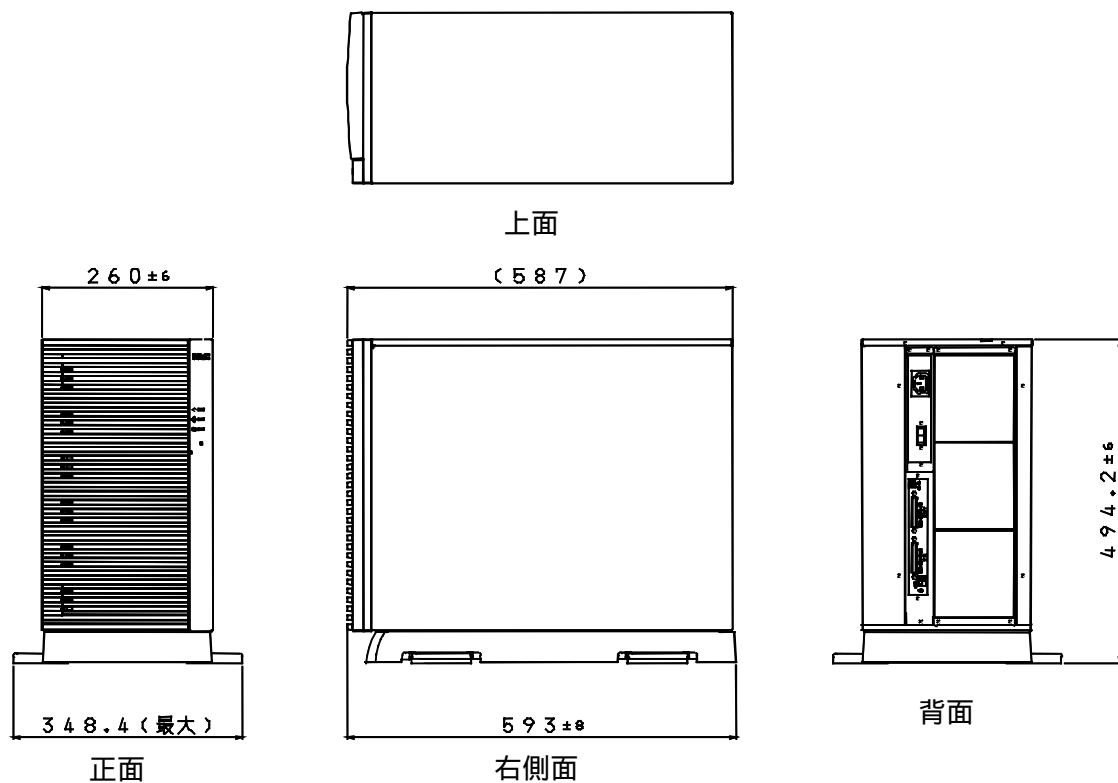
( N8590-13 ) 筐体寸法 260\text{mm(W)} \times 587\text{mm(D)} \times 494.2\text{mm(H)}
