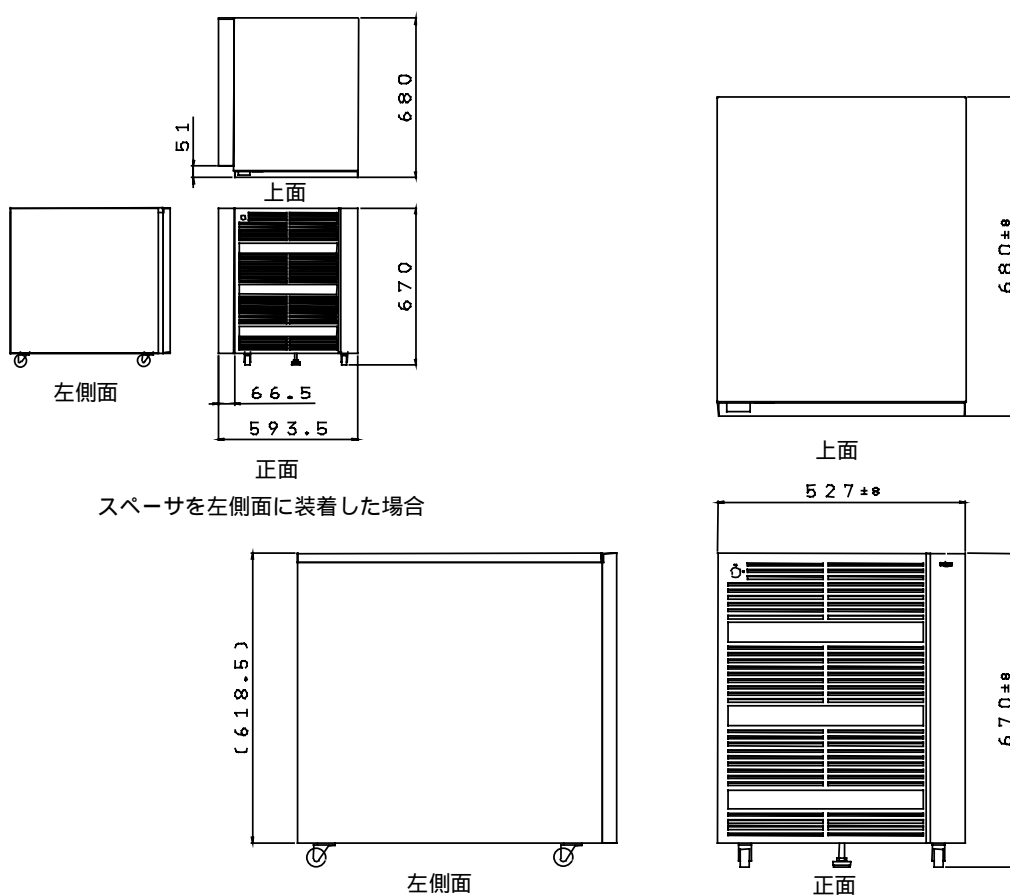
( N8590-14 ) 筐体寸法 527\text{mm(W)} \times 680\text{mm(D)} \times 670\text{mm(H)}
