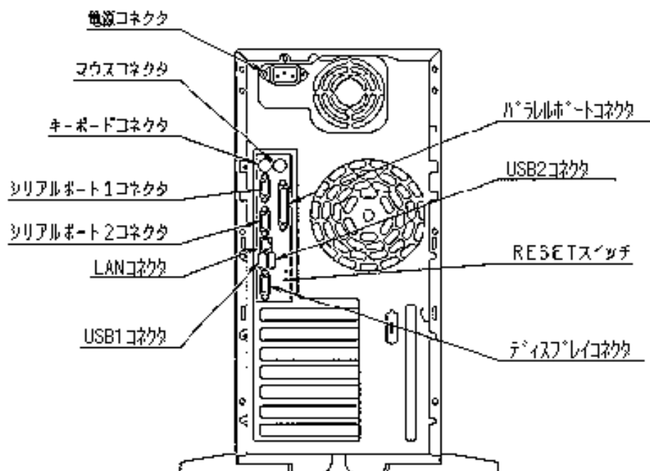
背面図
