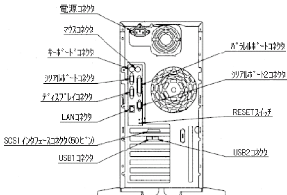
背面図
