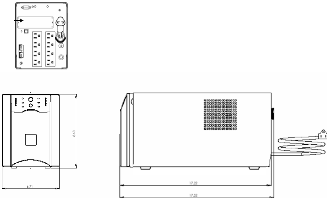
N8180-45A/-46A 外觀圖 170mm(W) × 445mm(D) × 219mm(H)
