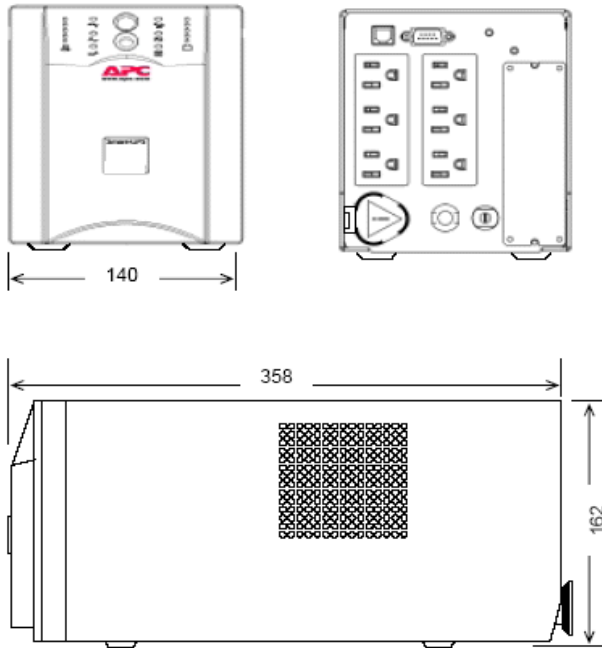
N8180-49/49A/50 外觀圖 140mm(W) × 358mm(D) × 162mm(H)
