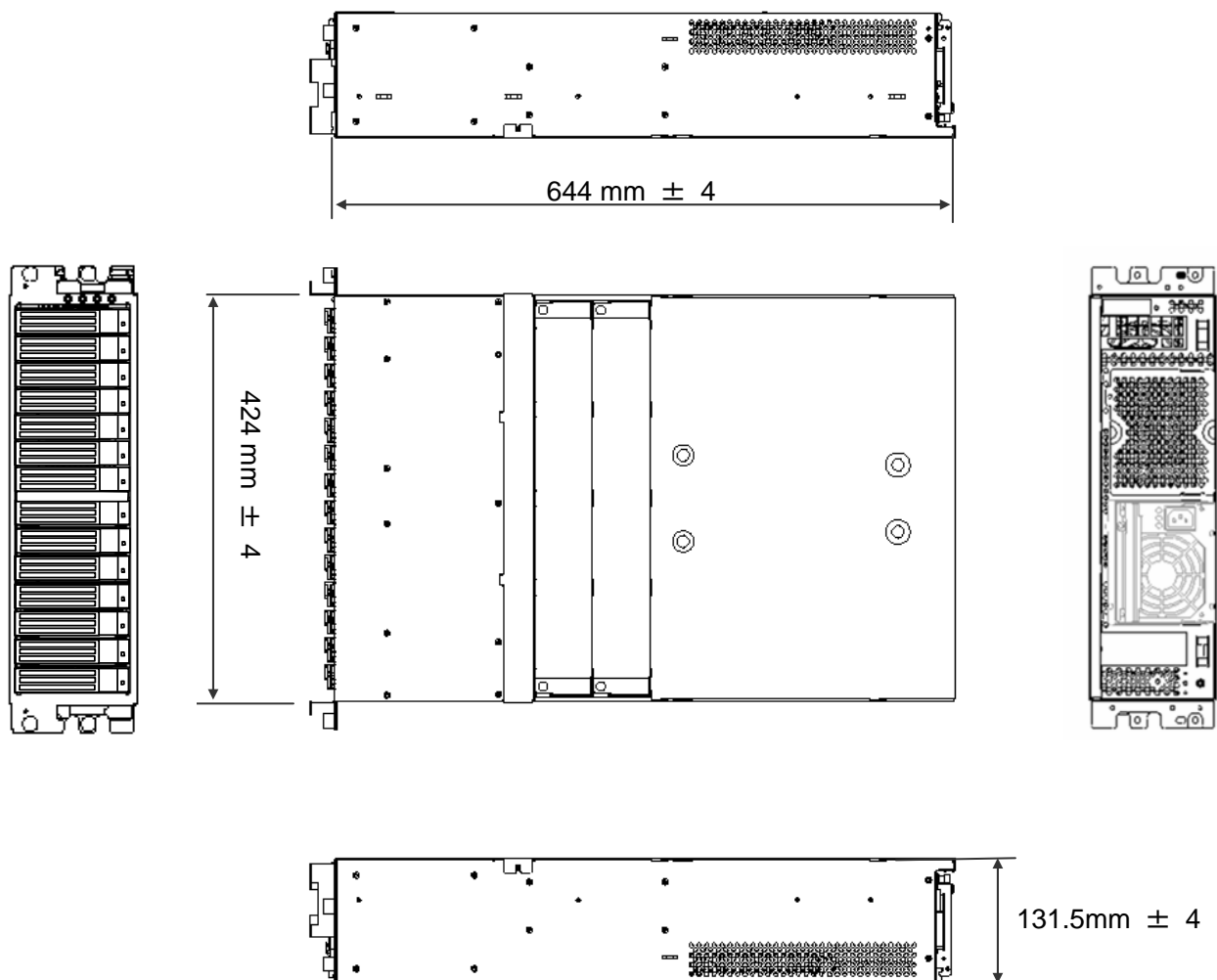
[N8141-39] 筐体寸法 424 mm(W) × 644 mm(D) × 131.5 mm(H)
