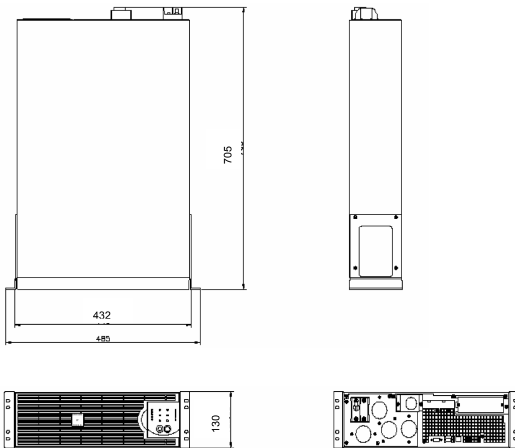
裏面図
