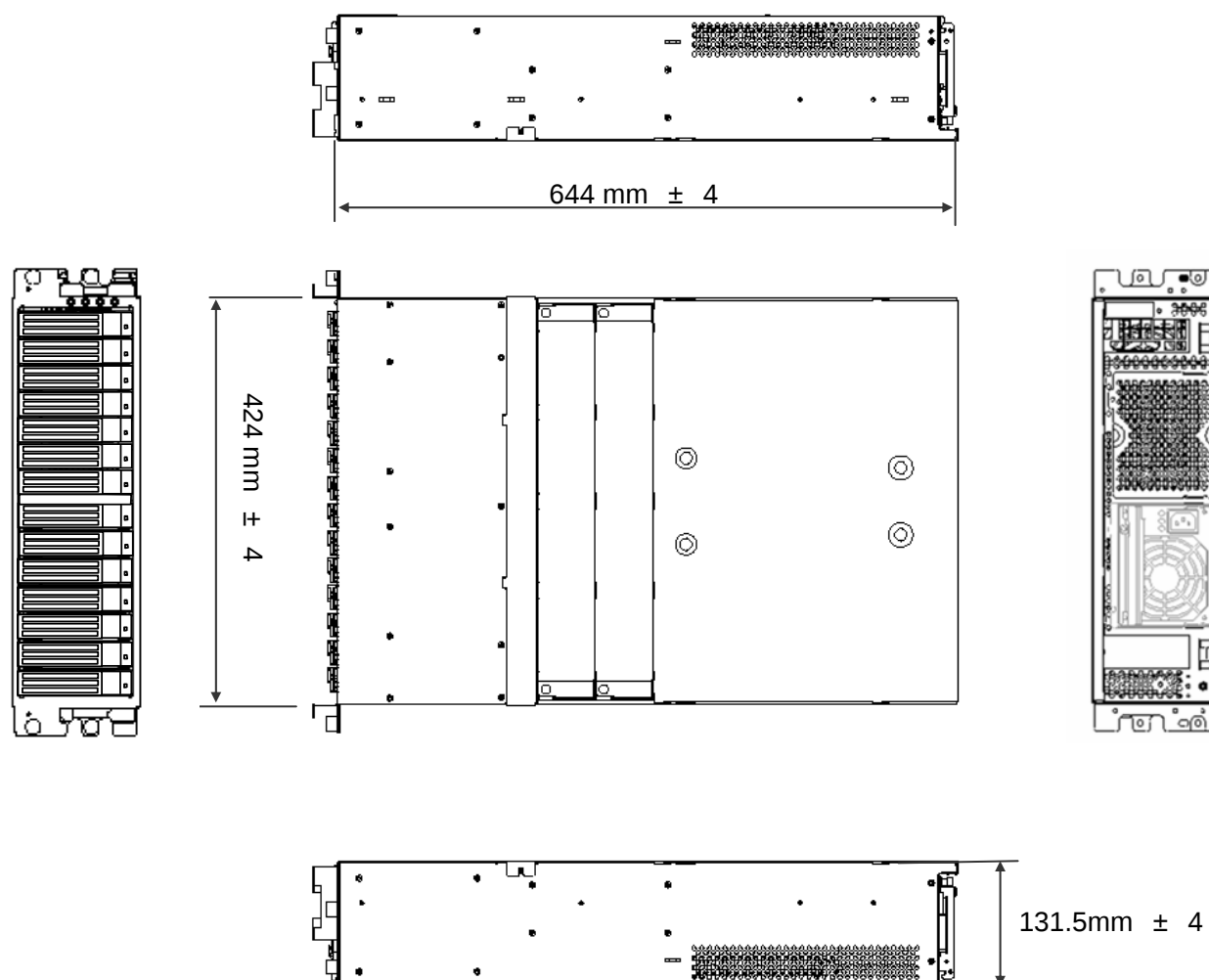
[N8141-36] 筐体寸法 424 mm(W) × 644 mm(D) × 131.5 mm(H)
