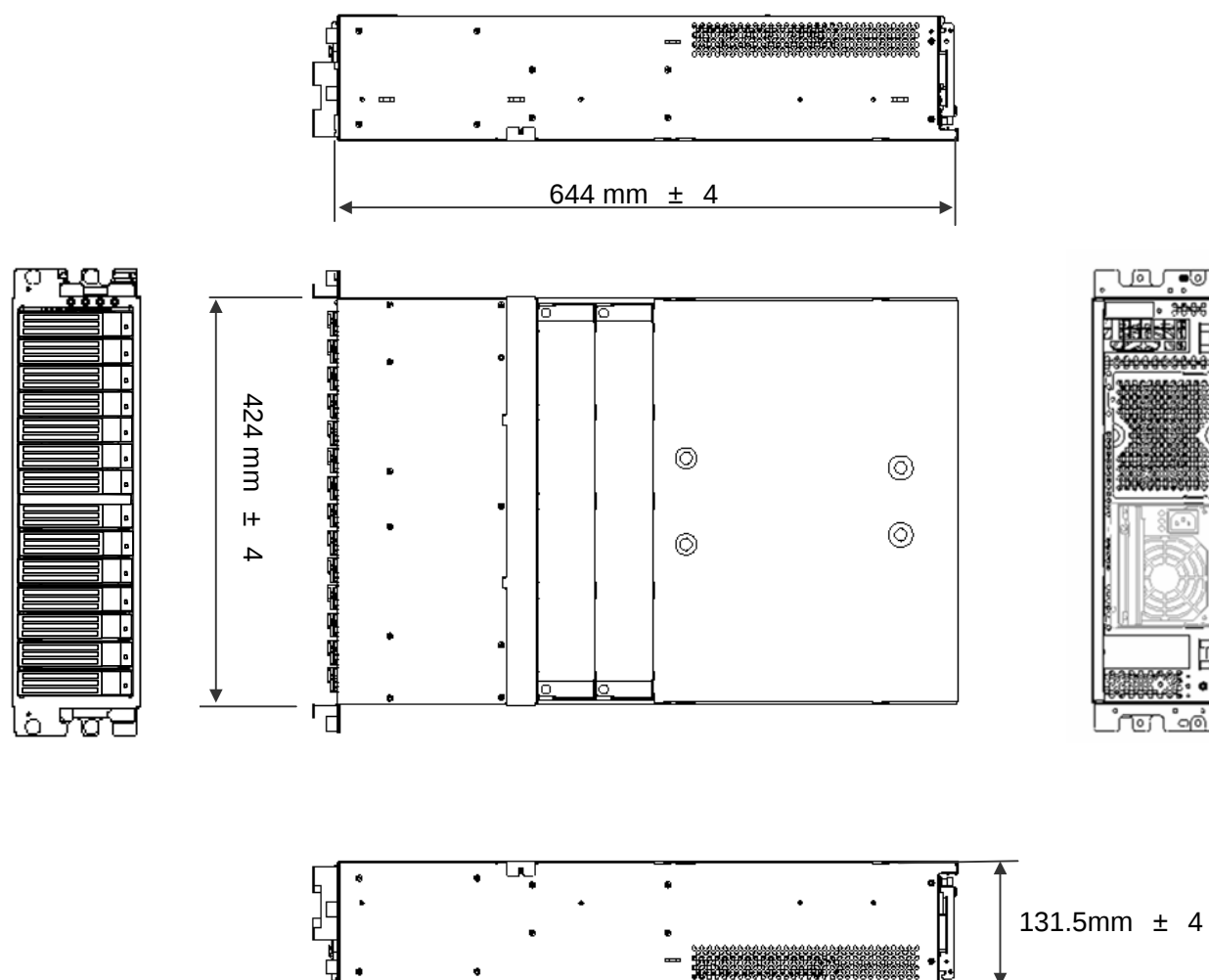
[N8141-36] 筐体寸法 424\text{ mm(W)} \times 644\text{ mm(D)} \times 131.5\text{ mm(H)}
