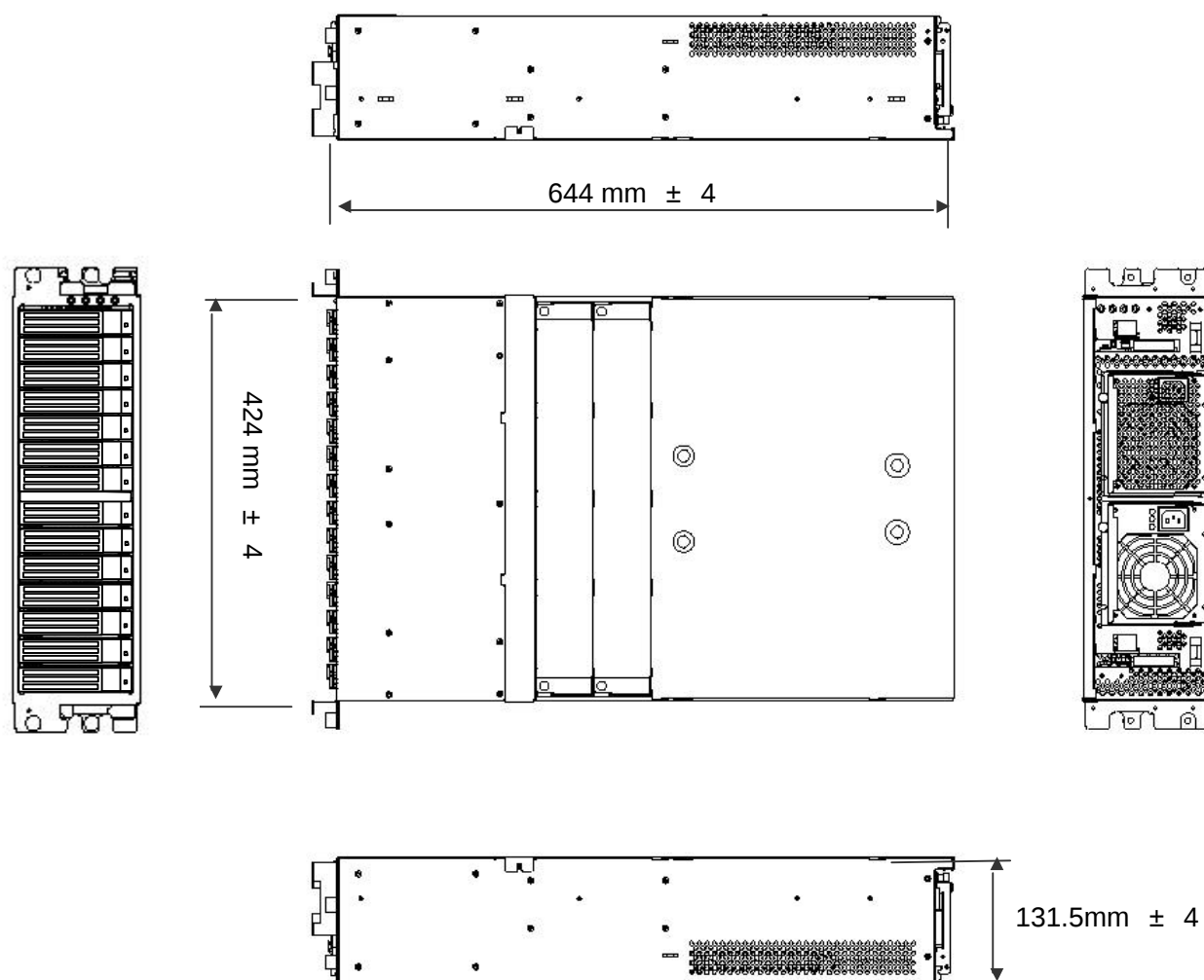
(N8141-32) 筐体寸法 424\text{ mm(W)} \times 644\text{ mm(D)} \times 131.5\text{ mm(H)}
