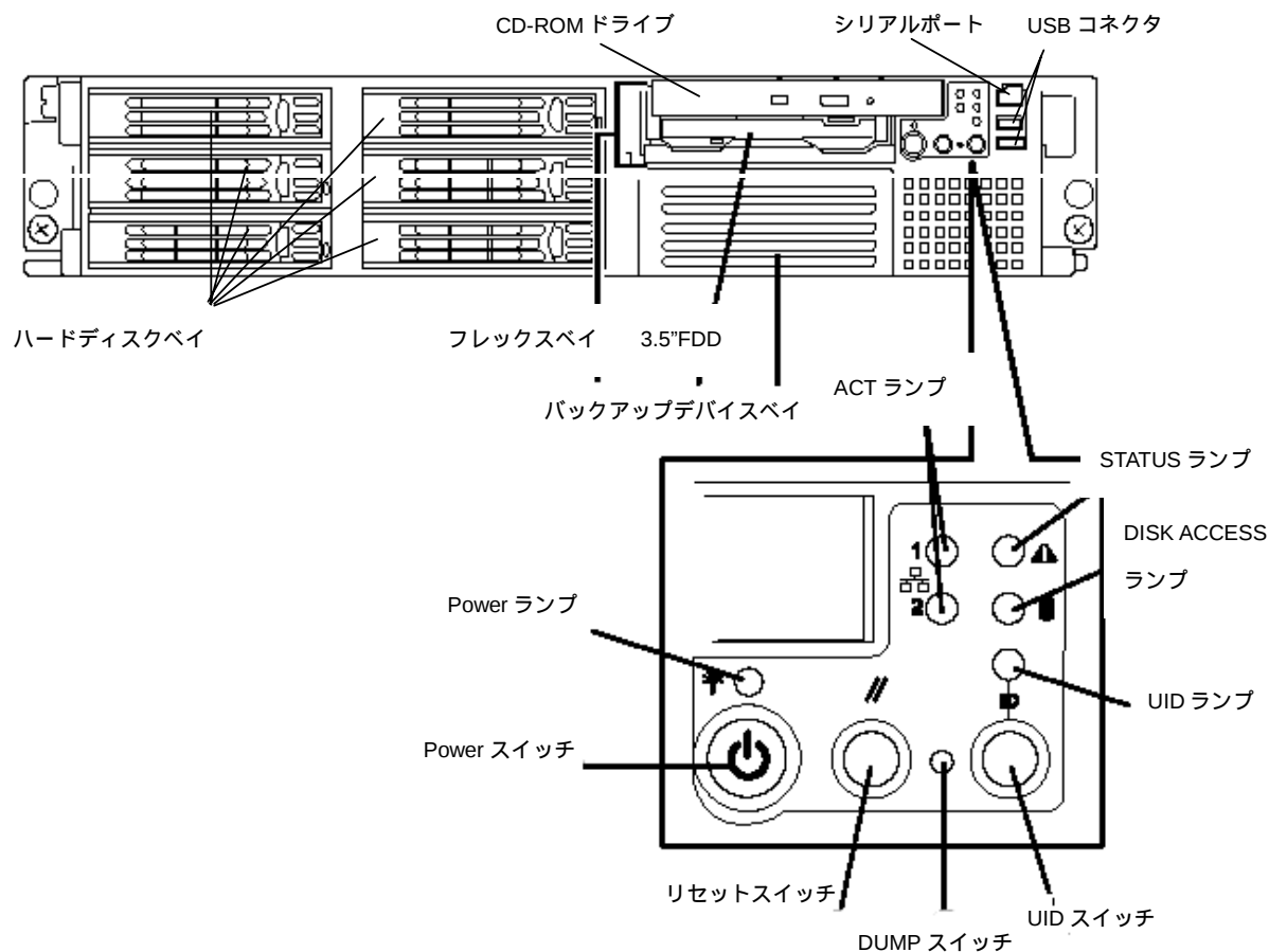
背面図
