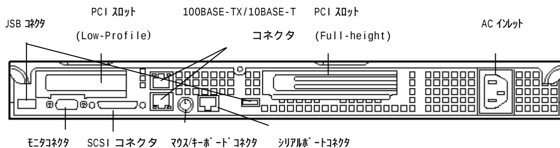
背面図
