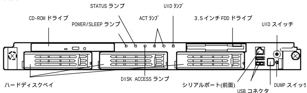
正面図
