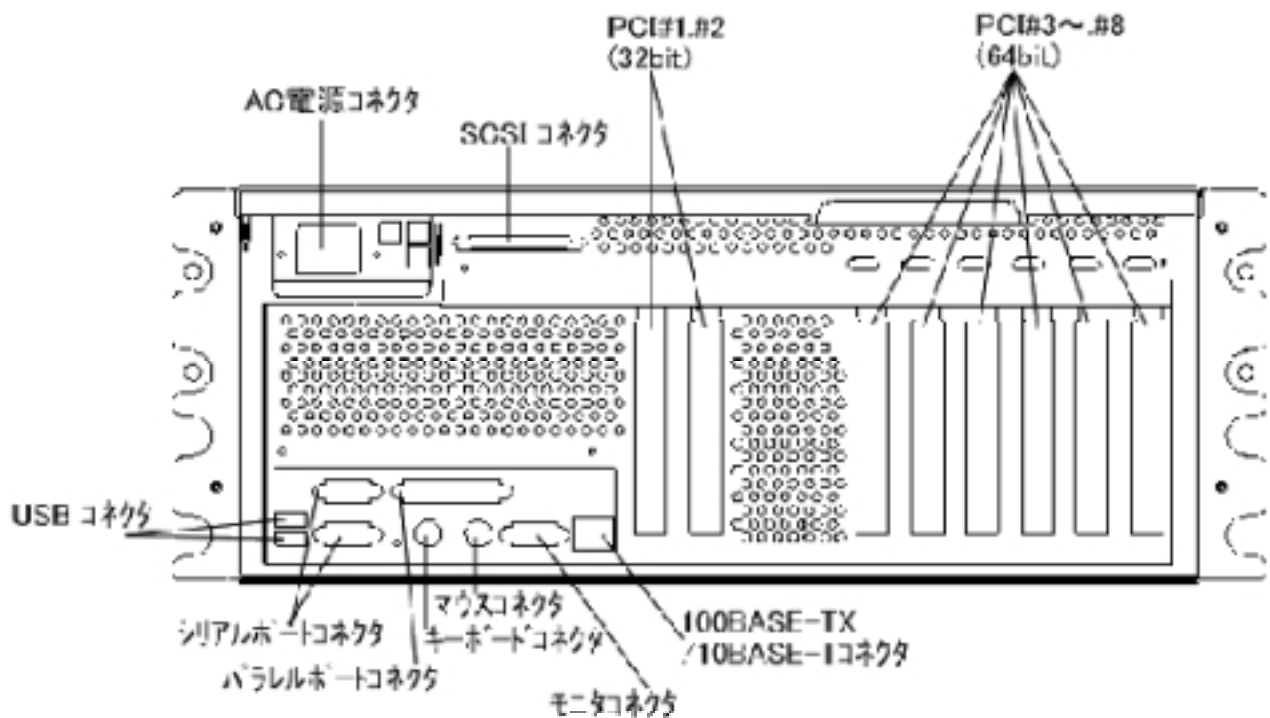
背面図
