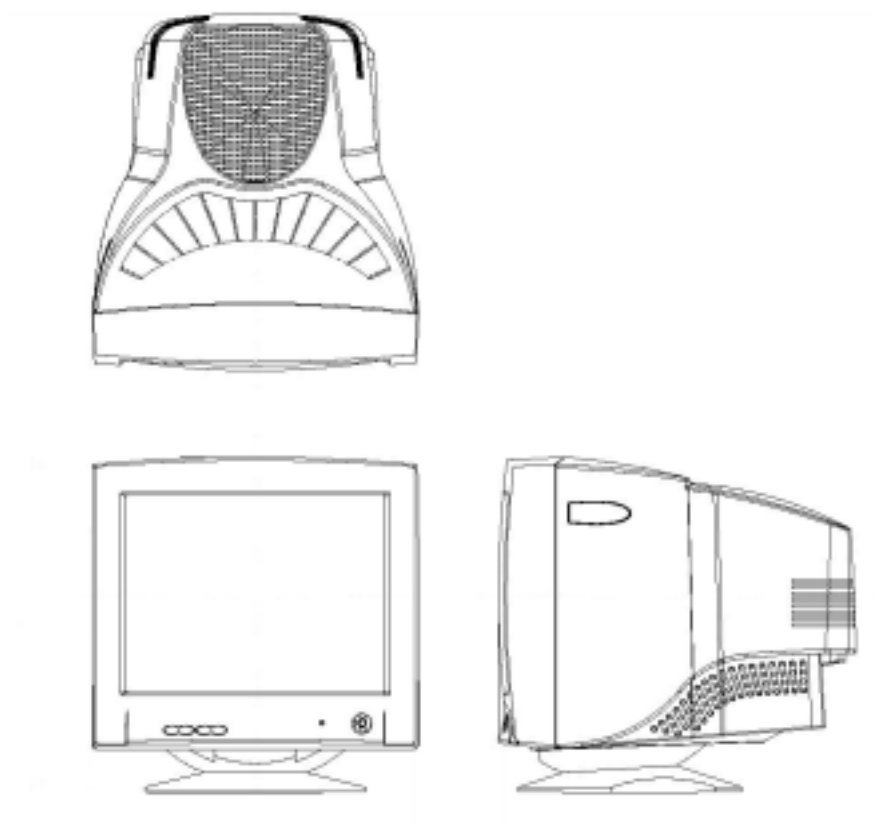
(N8171-30) 筐体寸法 363mm(W) × 398mm(D) × 374mm(H)
