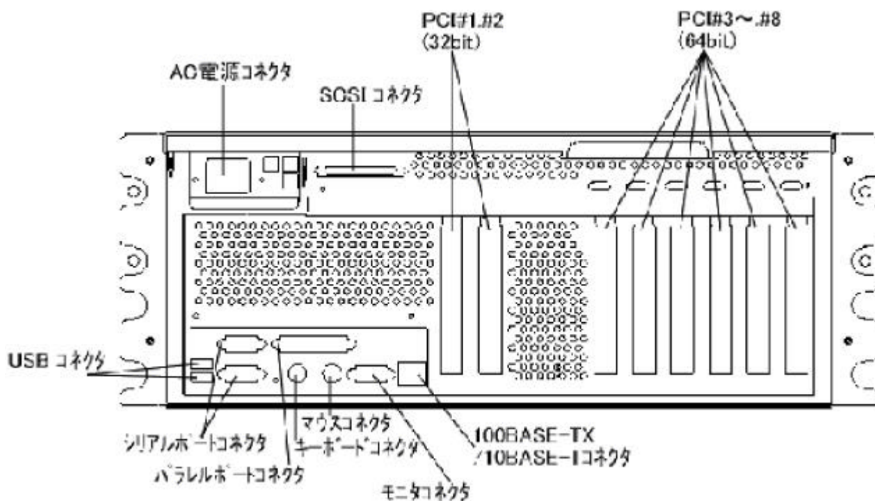
背面図
