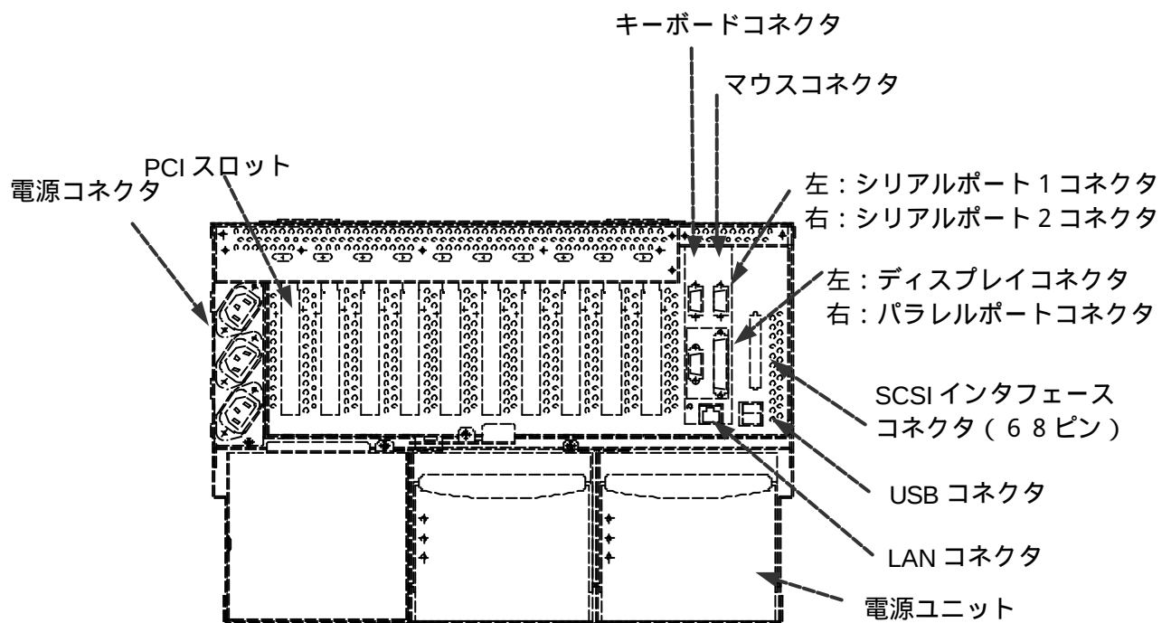
背面図
