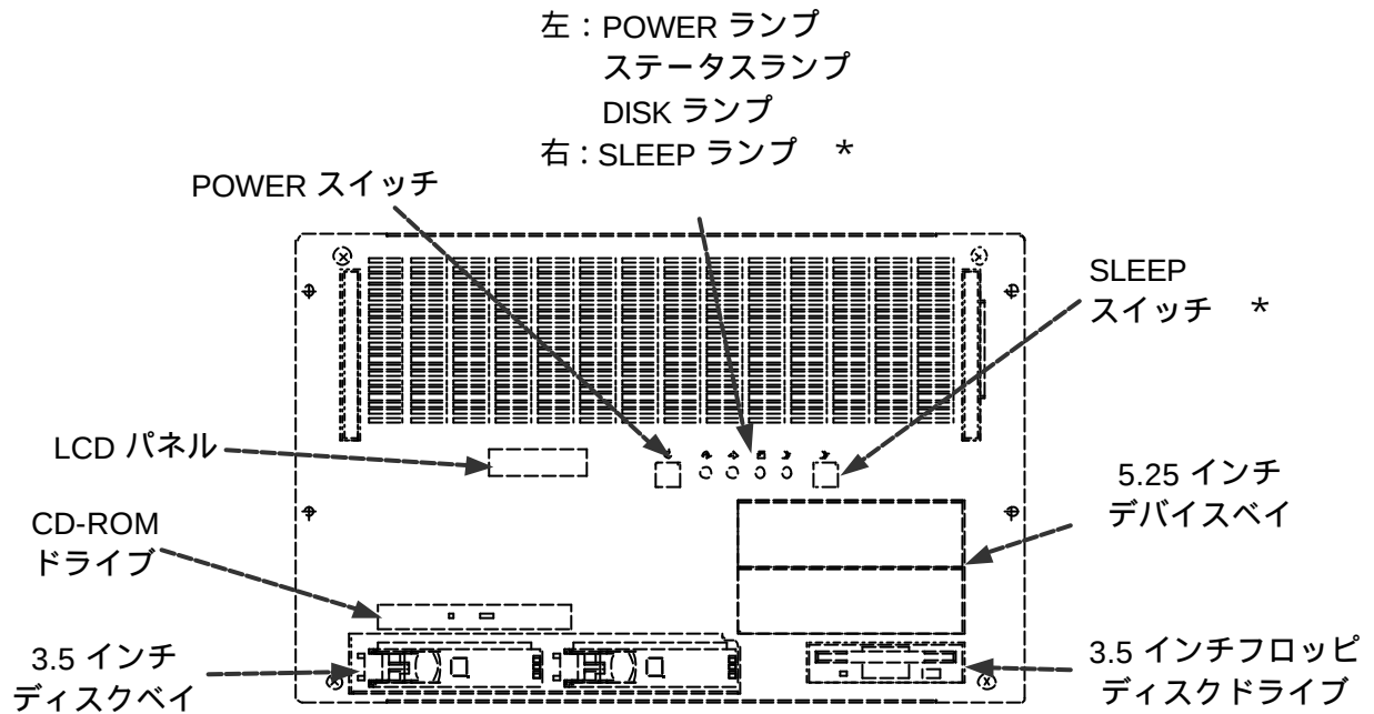
背面図
