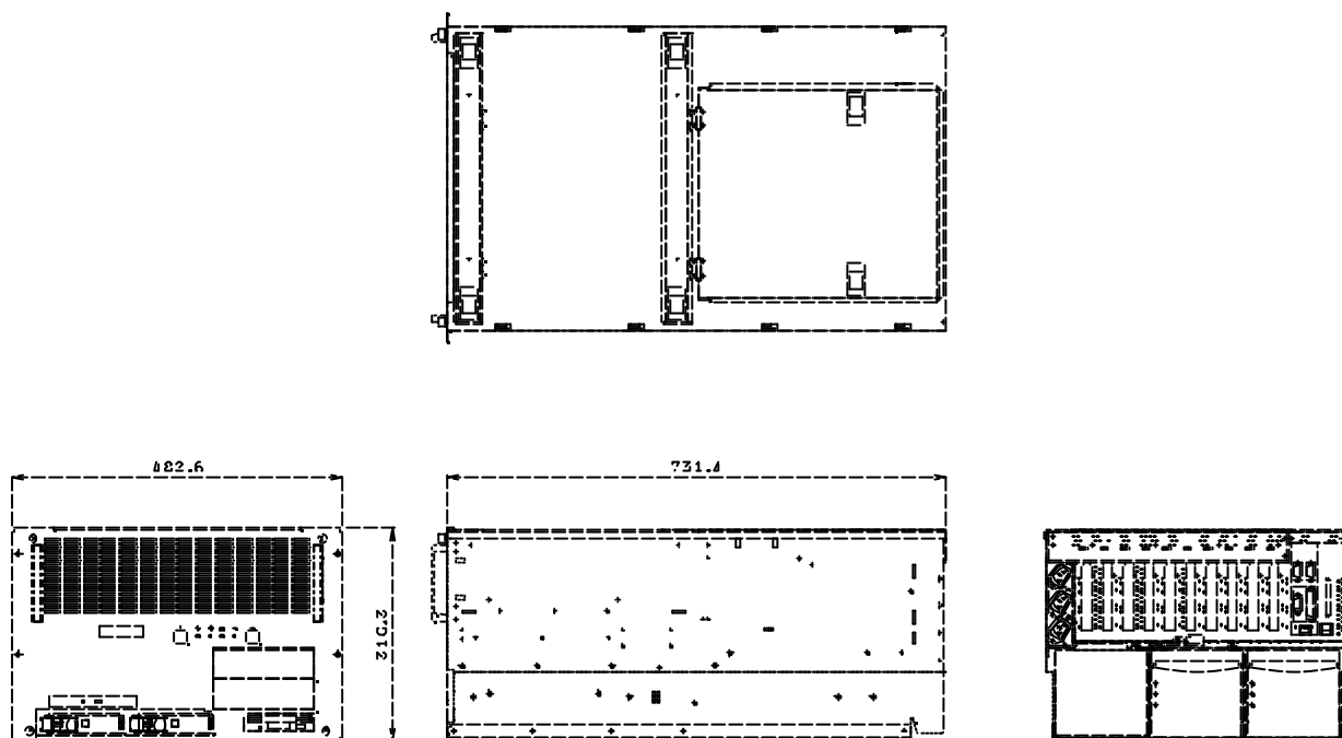
外形寸法 483(W)x735(D)x310(H) mm
