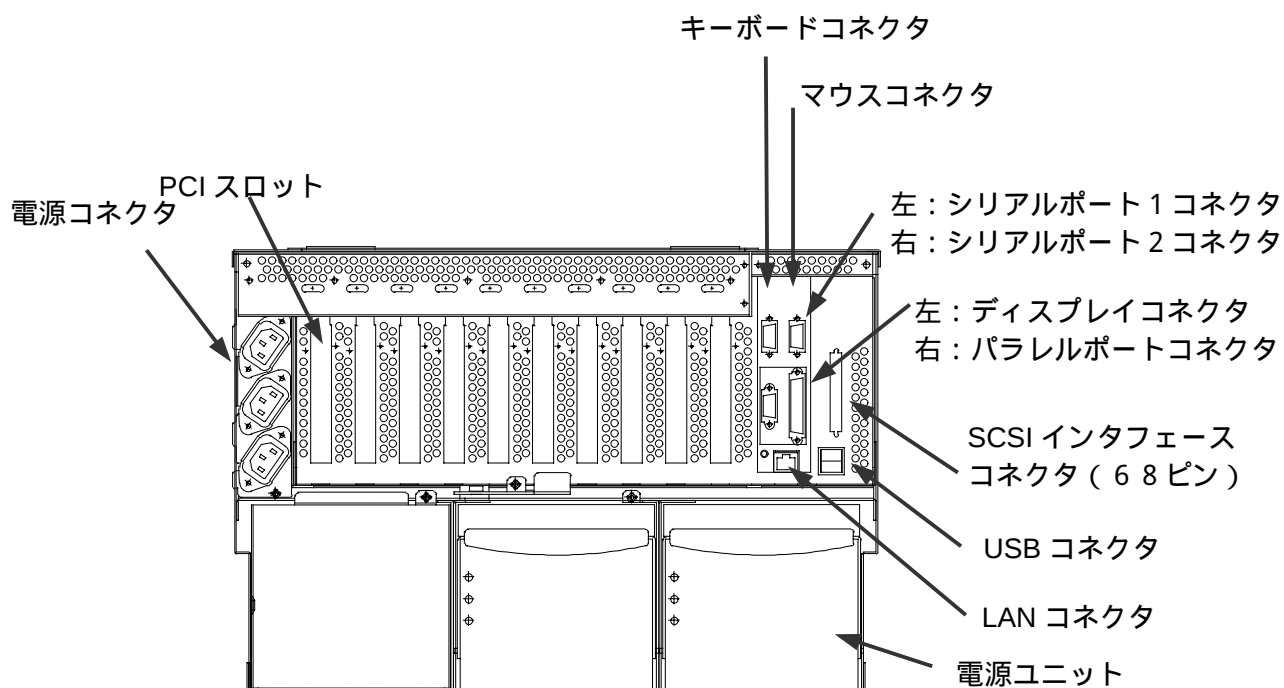
背面図
