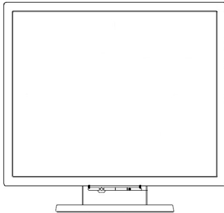
(N8171-43/43W) 筐体寸法 412.5(W) × 220(D) × 386.5~496.5(H)mm
