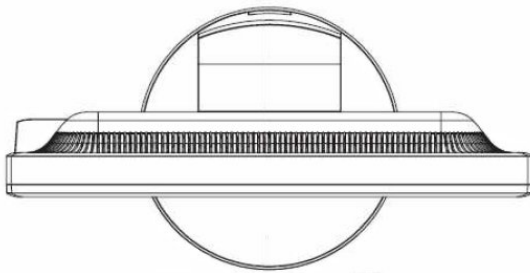
(N8171-43/43W) 筐体寸法 412.5(W) × 220(D) × 386.5~496.5(H)mm
