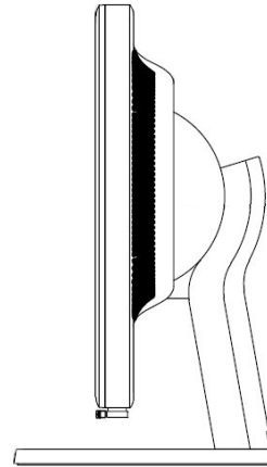
(N8171-43/43W) 筐体寸法 412.5(W) × 220(D) × 386.5~496.5(H)mm
