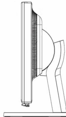
(N8171-44/44W) 筐体寸法 442(W) × 220(D) × 388.5~498.5(H)mm
