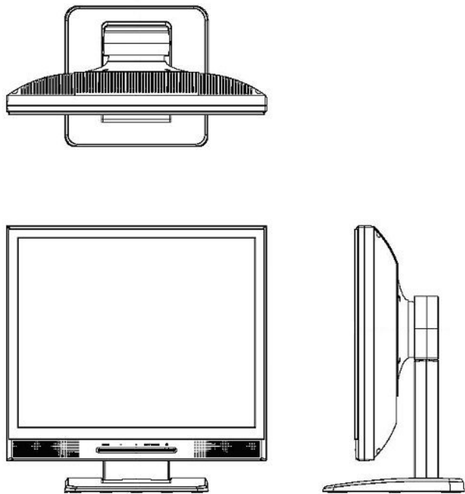
(N8171-40) 筐体寸法 418(W)×277(D)×427~497(H)mm
