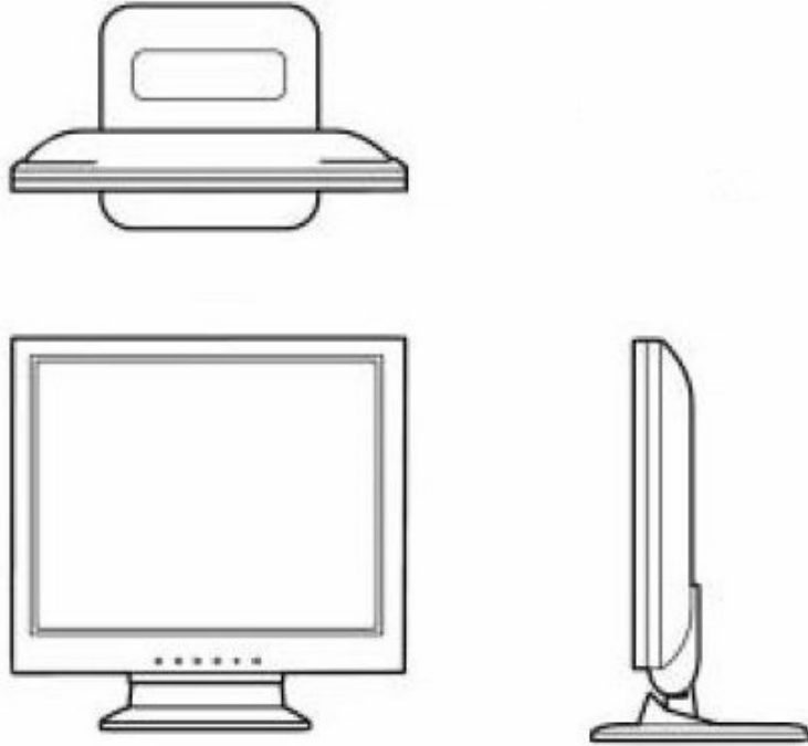
(N8171-42) 筐体寸法 339(W)×187(D)×322(H)mm
