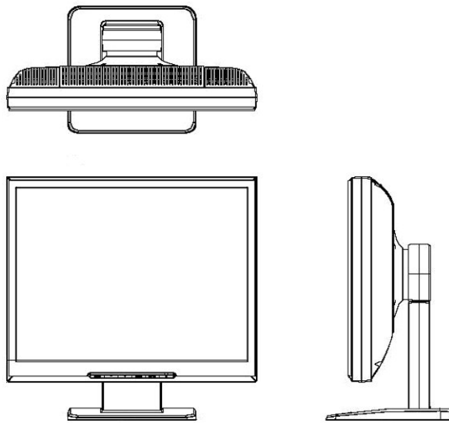
(N8171-41) 筐体寸法 446(W)×227(D)×435~505(H) mm
