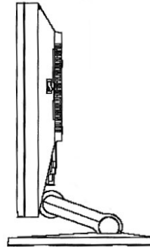
(N8171-39) 筐体寸法 381(W)×222(D)×365~412(H)mm
