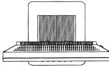
(N8171-34) 筐体寸法 343(W)×170(D)×308(H)mm
