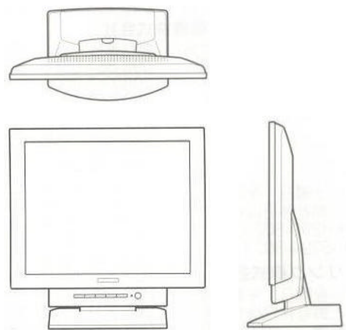
(N8171-27) 筐体寸法 377mm(W) × 180mm(D) × 390mm(H)
