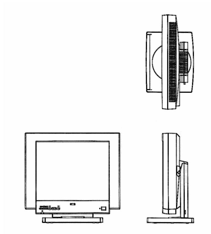
(N7832-46) 筐体寸法 516mm(W) × 255mm(D) × 487mm(H)
