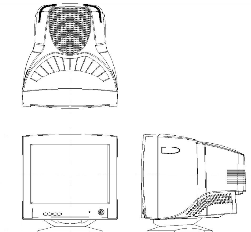
(N8171-30) 筐体寸法 363mm(W) × 398mm(D) × 374mm(H)
