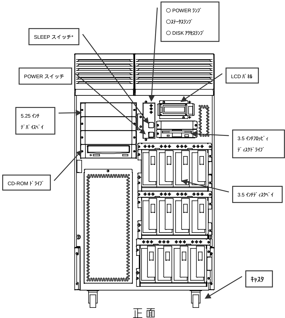
正面図
