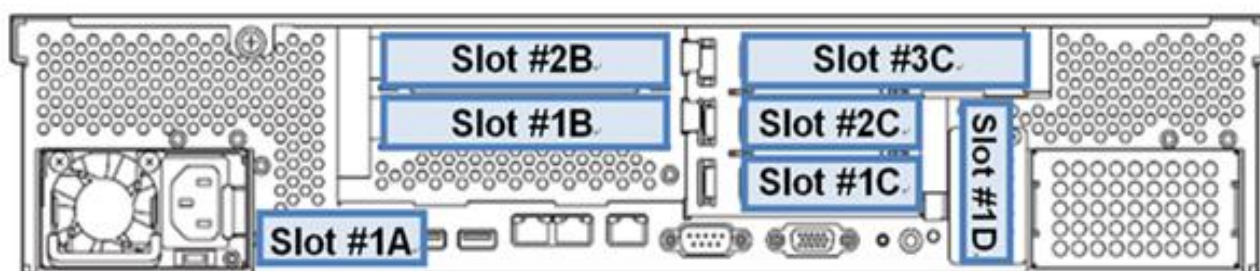
Express5800/R120d-2M、Express5800/R120e-2M 拡張スロット対応図
