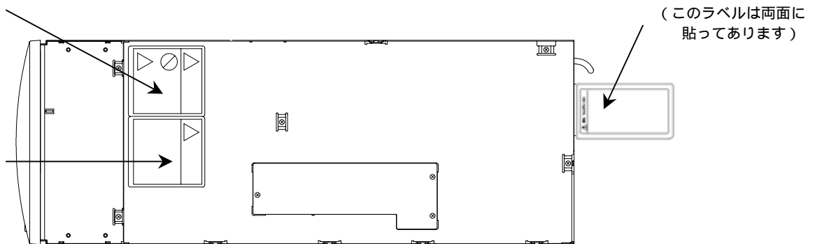
図 N8160-62 LT0 集合型（ラックマウント用）ラベル貼付位置
