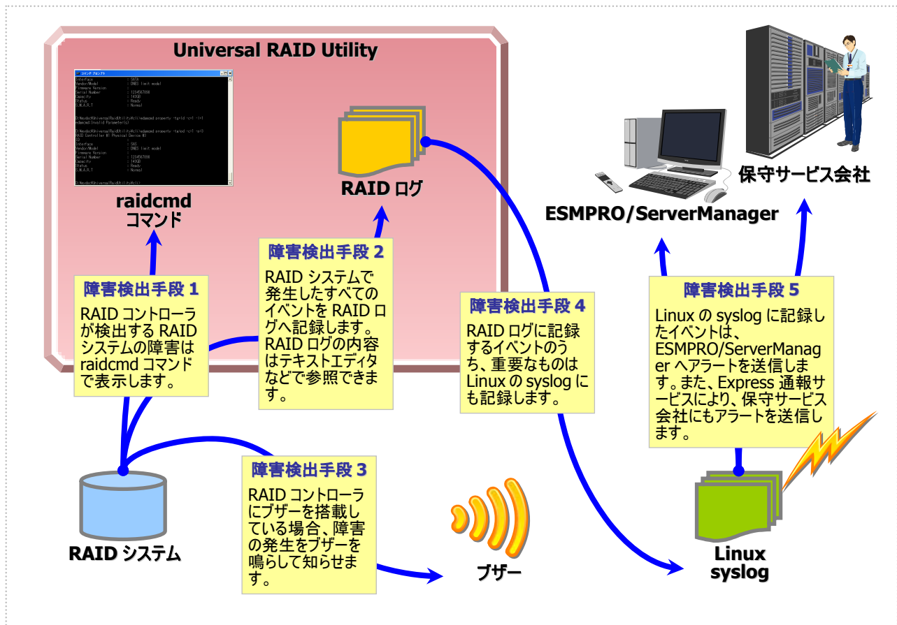
図 9 RAID システムの障害監視イメージ
